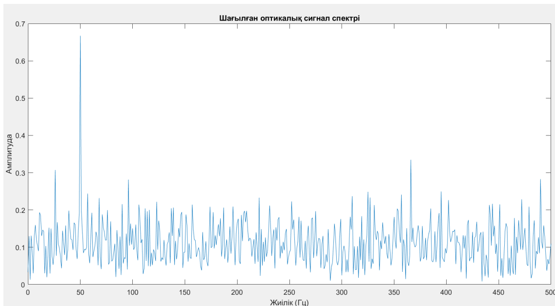
6-сурет. – Шағылысқан оптикалық сигналдың спектрі.
