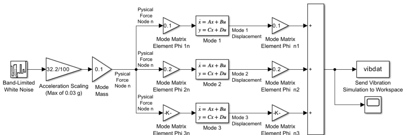
3-сурет. – Simulink бағдарламасындағы сұлба.
