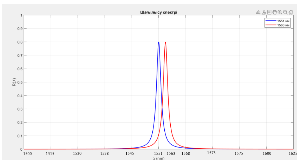
5-сурет. – 1551 НМ және 1566 НМ толқын ұзындығы үшін шағылысу спектрі.
