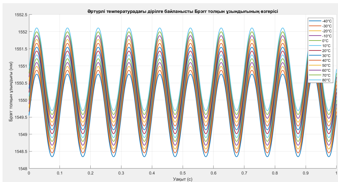
8-сурет. – Әртүрлі температурадағы дірілге байланысты Брэгг толқын ұзындығының өзгерісі.
