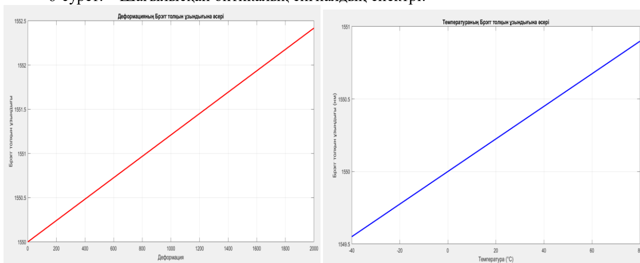
7-сурет. – Деформацияланған температураның Брэгг толқын ұзындығына әсері.
