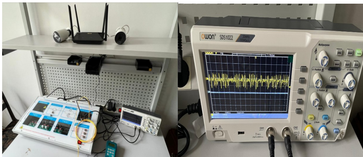
1-сурет. – Периметрді қорғауға арналған зертханалық қондырғы.
